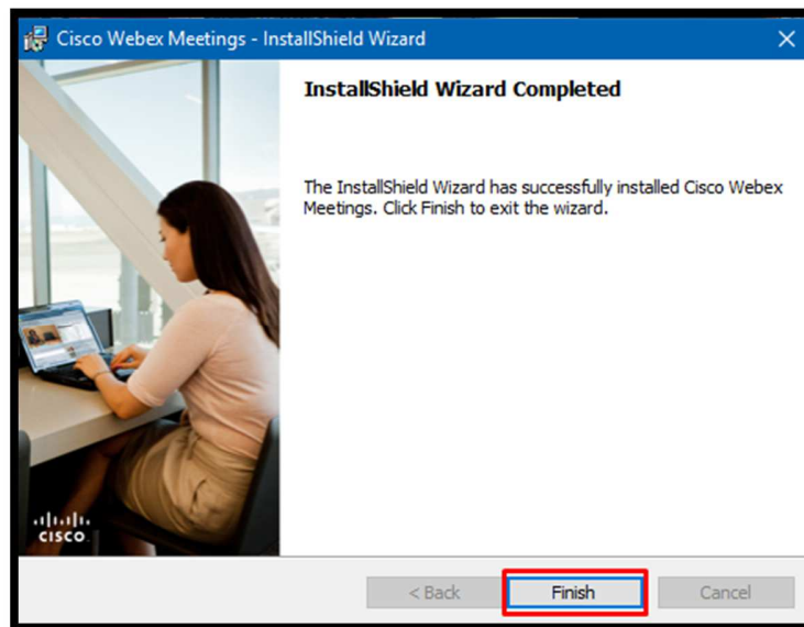
SLIKA 8 - ZAVRŠETAK INSTALACIJE
