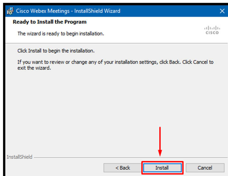
SLIKA 7 - POČETAK INSTALACIJE
