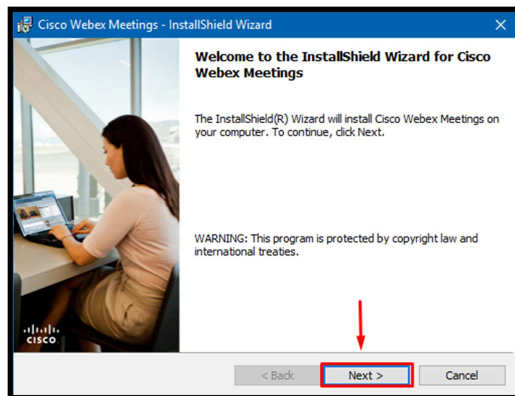
SLIKA 5 - PROCES INSTALACIJE
